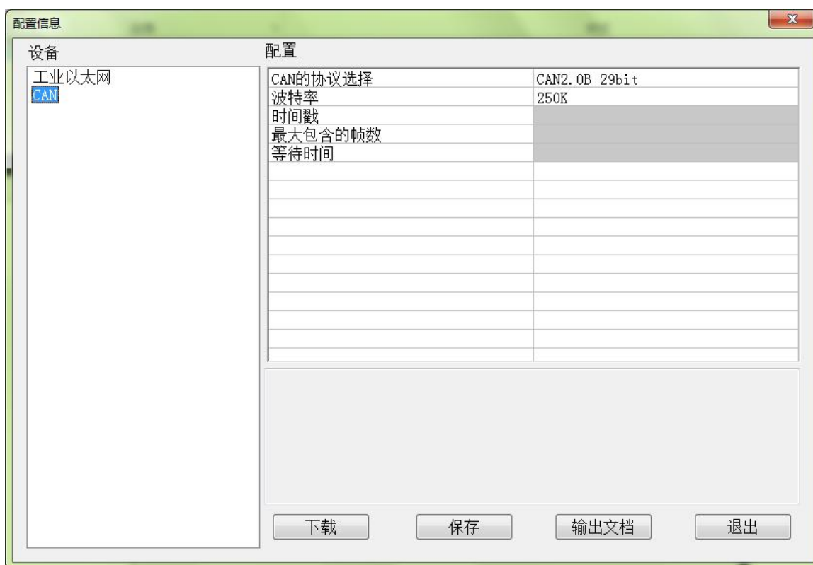
图 6 CAN 口配置信息
