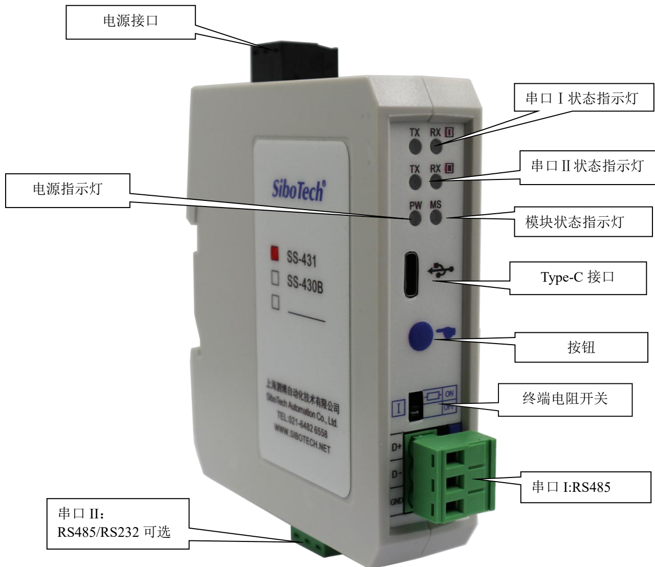
图 1 产品外观
